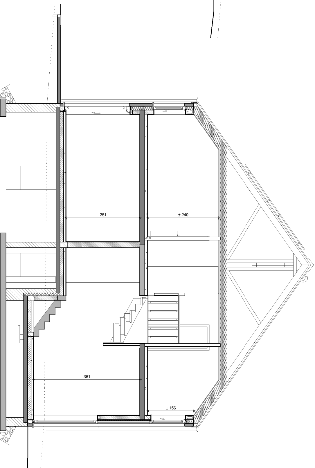
COUPE B-B
